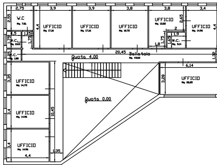
Planimetria UFFICI PRIMO PIANO - C.DA SAN NICOLA mq. 202,14
