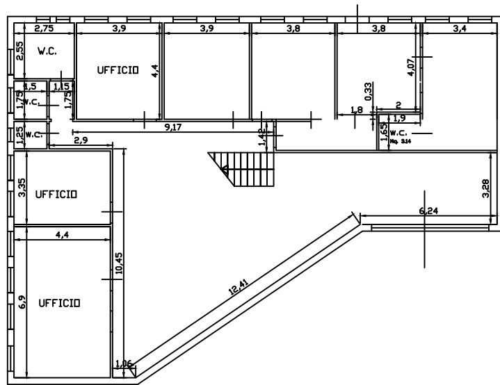
Planimetria UFFICI PIANO TERRA - C.DA SAN NICOLA mq. 194,00
