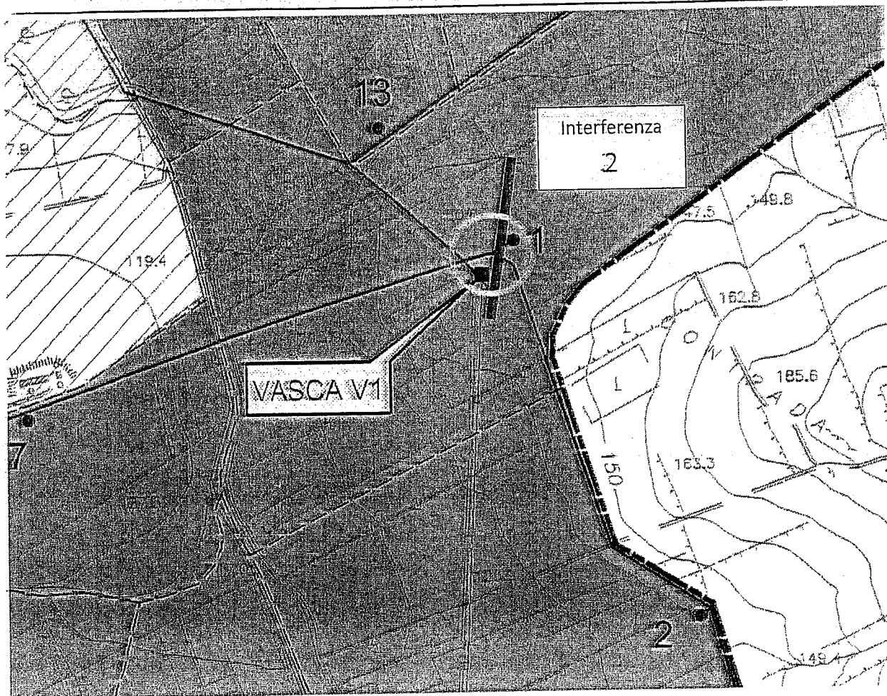
2 Zona prossima al gruppo di consegna 1 - interferenza con DN 700 acciaio
